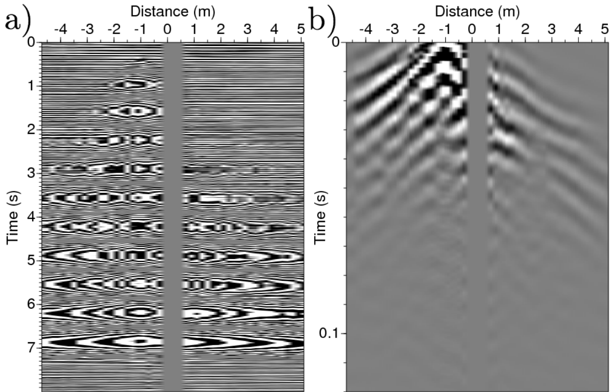
FIGURE 5.28 – Sismogrammes obtenus pour un tir en surface réalisé avec le pot vibrant commandé par un signal chirp et situé à 1.3m à l'Est de la cheminée (a); intercorrélation de ce signal avec le sismogramme du capteur de référence (b)
